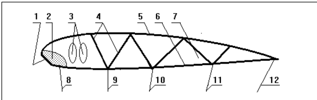
Рис. 47. Разрез купола параплана по силовой нервюре.
