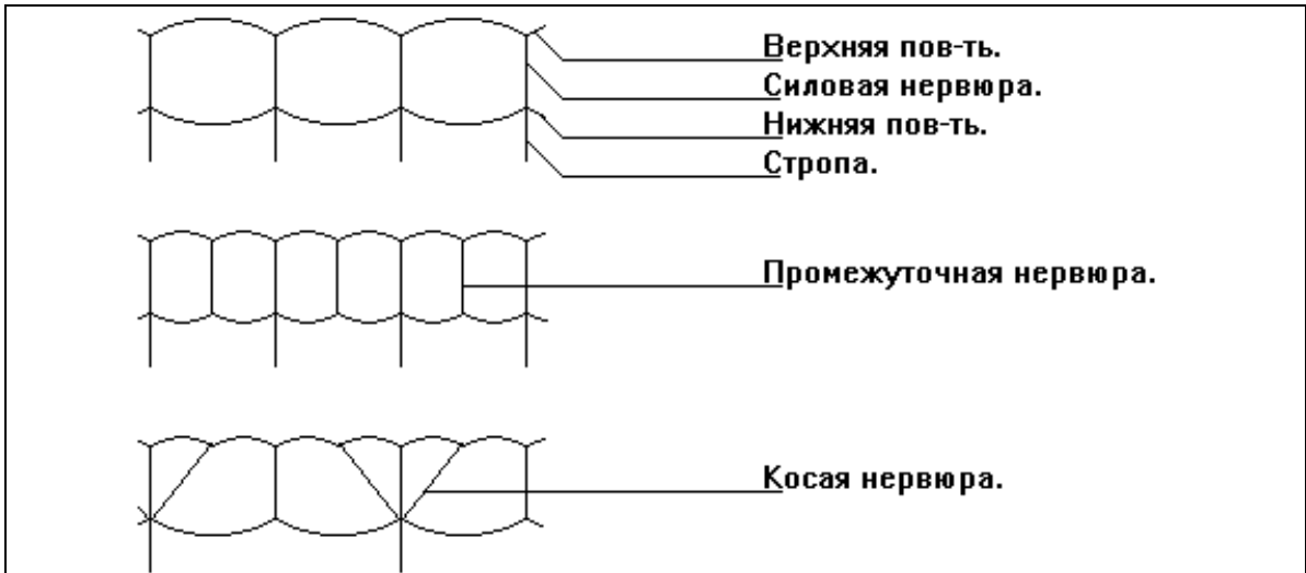
Рис. 48. Виды нервюр.
