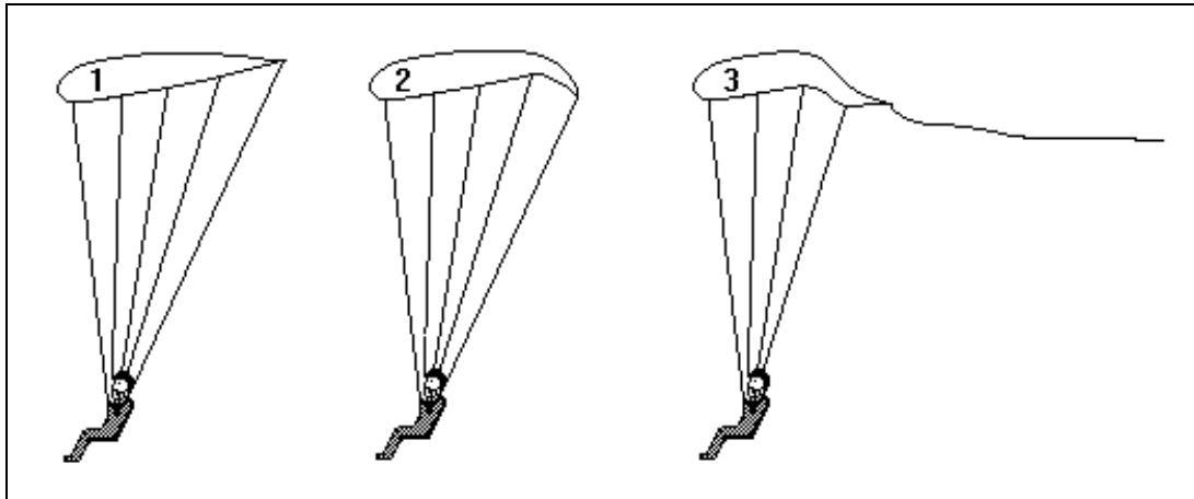
Рис. 62. Аэродинамический способ управления парашютом. 1 – планирование. 2 – управление клевантой. 3 - управление за 4-й ряд строп при обрыве стропы управления.
