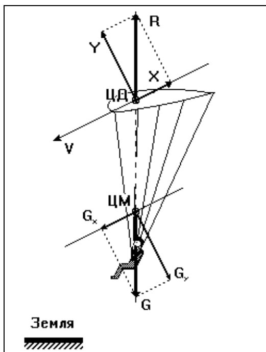
Рис. 61. Силы, действующие на парашютан в прямолинейном полете. ЦД – центр давления. ЦМ – центр масс. R – полная аэродинамическая сила. Y – подъемная сила. X – сила аэродинамического сопротивления. G – сила тяжести. V – воздушная скорость.
