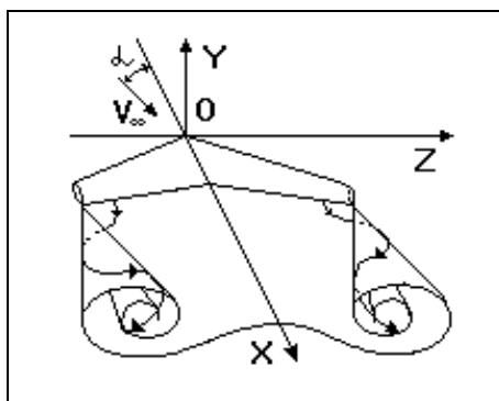
Рис. 40. Образование вихрей на законцовках крыла.
