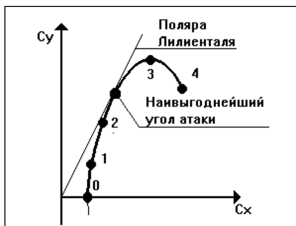
Рис. 25. Поляра крыла.
