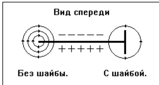
Рис. 43. Уменьшение индуктивного сопротивления с помощью концевых шайб.
