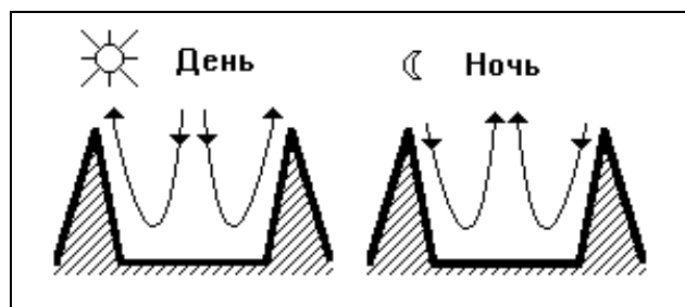
Рис. 108. Горные бризы.
