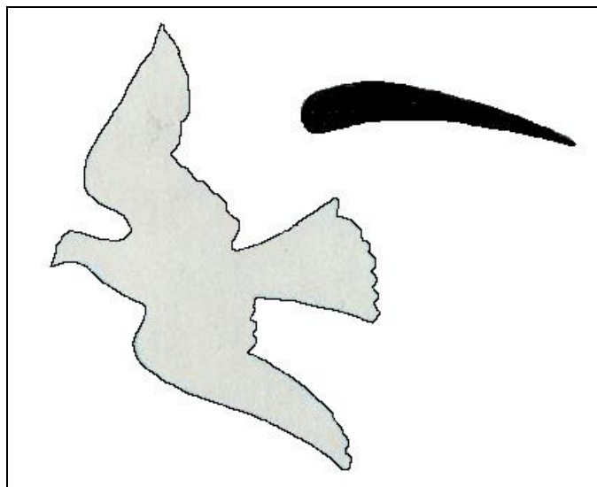
Рис. 34. Крыло птицы.
