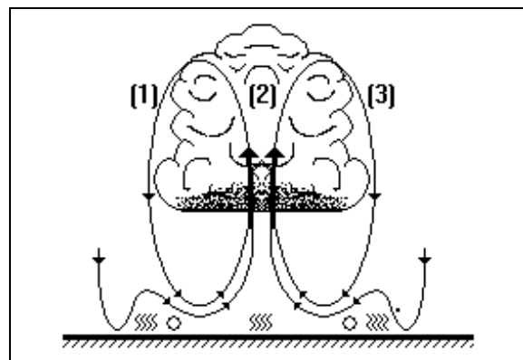
Рис. 137. Кучевое облако превращается в мощное кучевое.
